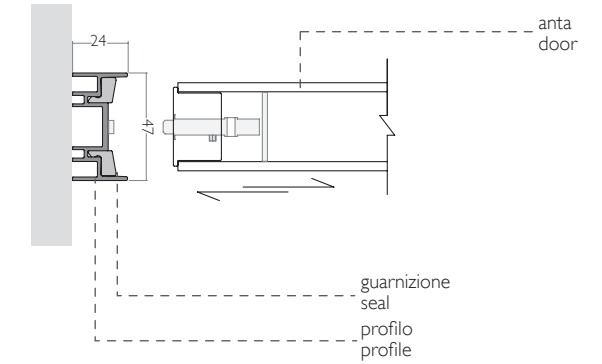
Profilo di battuta per serratura / Door striker profile for lock Versione binari a soffitto, a soffitto - cartongesso, con trave sospesa. Ceiling, plasterboard ceiling and hanging rail version.
