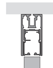
Binario a soffitto / Ceiling rail
