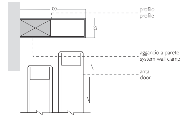
Profilo di battuta laterale / Side door striker profile Versione binari a parete 2 vie. 2 ways wall rail version.
