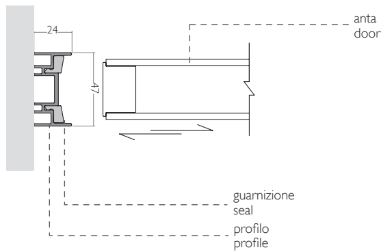
Profilo di battuta frontale / Front door striker profile Versione binari a soffitto, a soffitto - cartongesso, con trave sospesa. Ceiling, plasterboard ceiling and hanging rail version.
