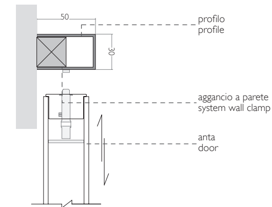
Profilo di battuta laterale per serratura / Side door striker profile for lock Versione binari a parete 1 via. 1 wall rail version.
