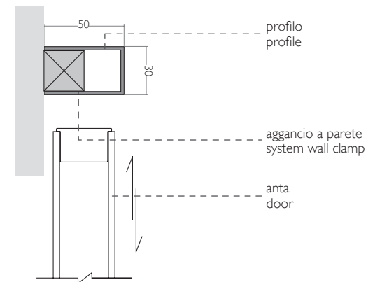
Profilo di battuta laterale / Side door striker profile Versione binari a parete 1 via. 1 wall rail version.
