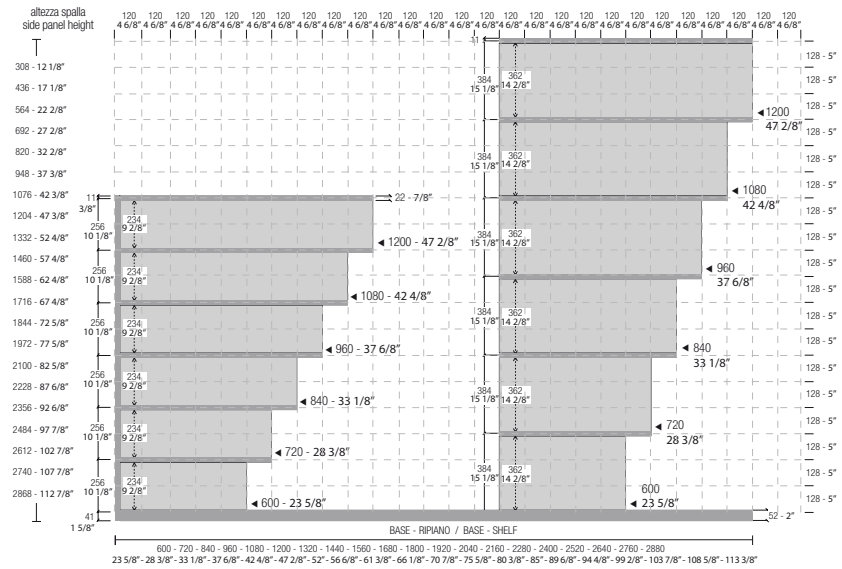
Griglia di sistema Grid system
