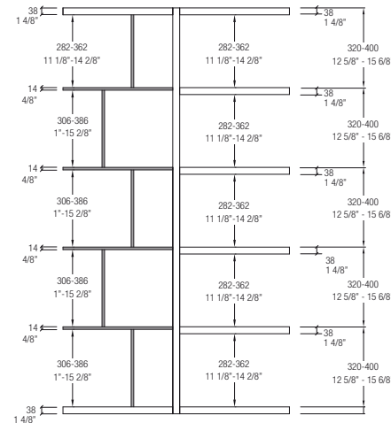
Altezza vani Compartment height
