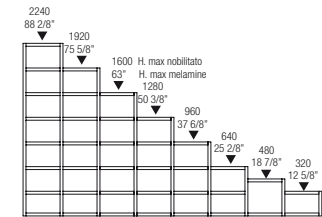
Altezza per moduli pensili Hights for hanging modules
