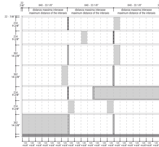
REGOLE DI COMPONIBILITA' COMPOSITIONS RULES
