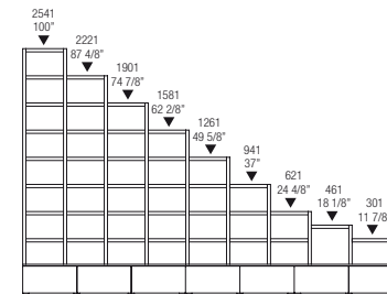
Altezza per moduli sopra su contenitori Heights for overhanging modules on containers
