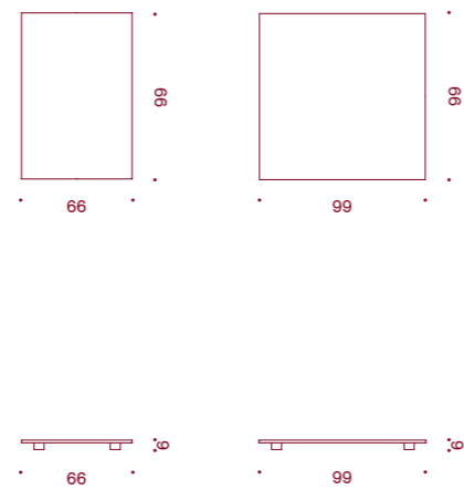
TAVOLINO H 6 SIDE TABLE H 6
